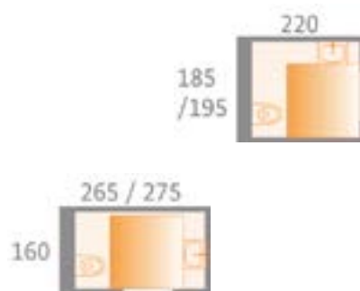
Flächenbedarf einer einseitig anfahrbaren Toilette mit Waschtisch oder Handwaschbecken
