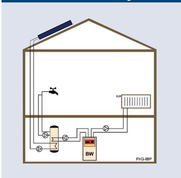
Abbildung 11: Schematische Darstellung einer Heizanlage mit solarer Warmwasserbereitung
