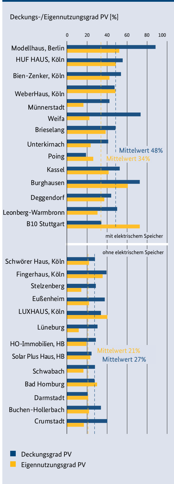
Abbildung 29: Eigennutzung und Deckung des Photovoltaikstroms für das erste Messjahr in den Ein- und Zweifamilienhäusern
